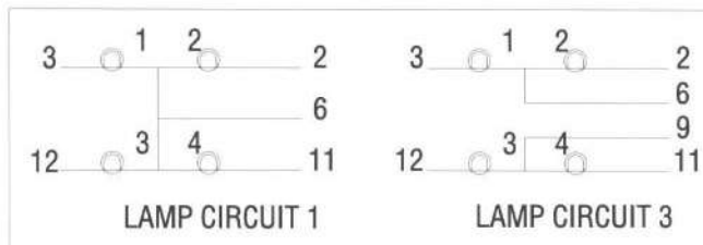
Lamp Circuits
