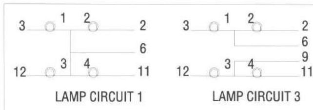
Lamp Circuits
